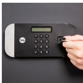
Ouverture de secours par clé à double panneton
