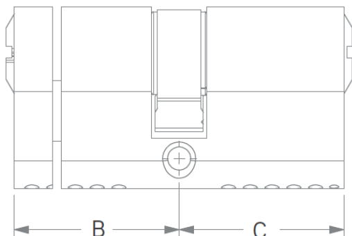
Fig.1 – cilindru dublu cu protecție anti-ruptură
